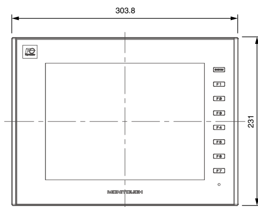
■正面部 Front view
