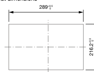
■パネルカット寸法 Panel cut dimensions
