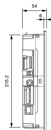
■側面部 Side view
