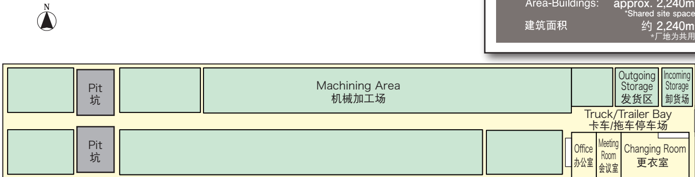
Layout 布局图
